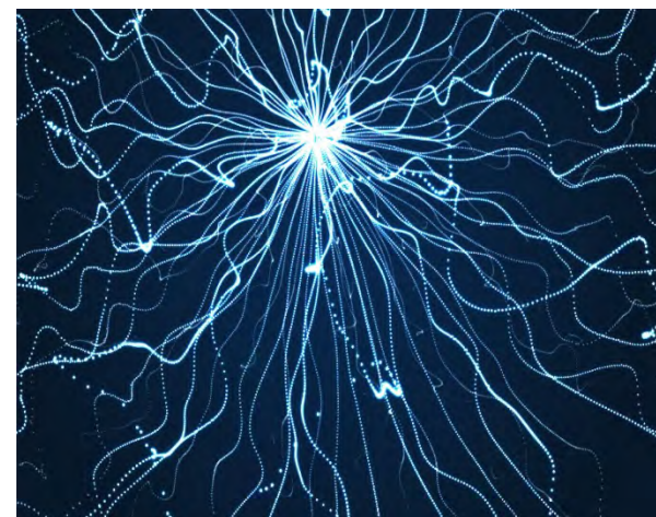
Ressources partagées
